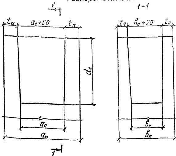
РАЗМЕРЫ СТАКАНА
