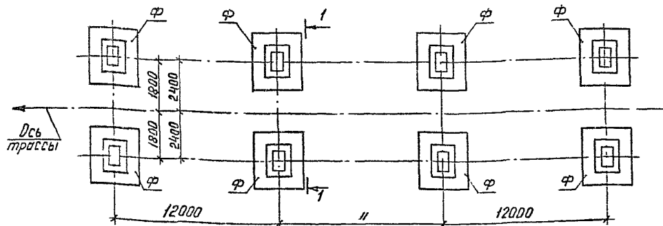
Схема №1
