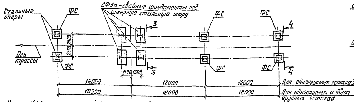
Схема №2
