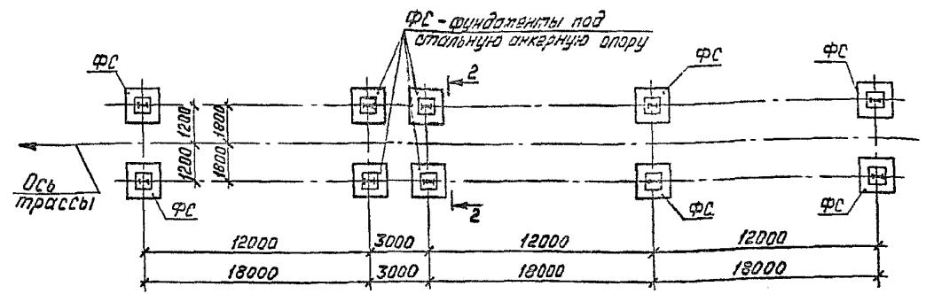
Схема № 2
