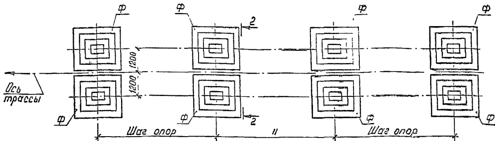
Схема №4
